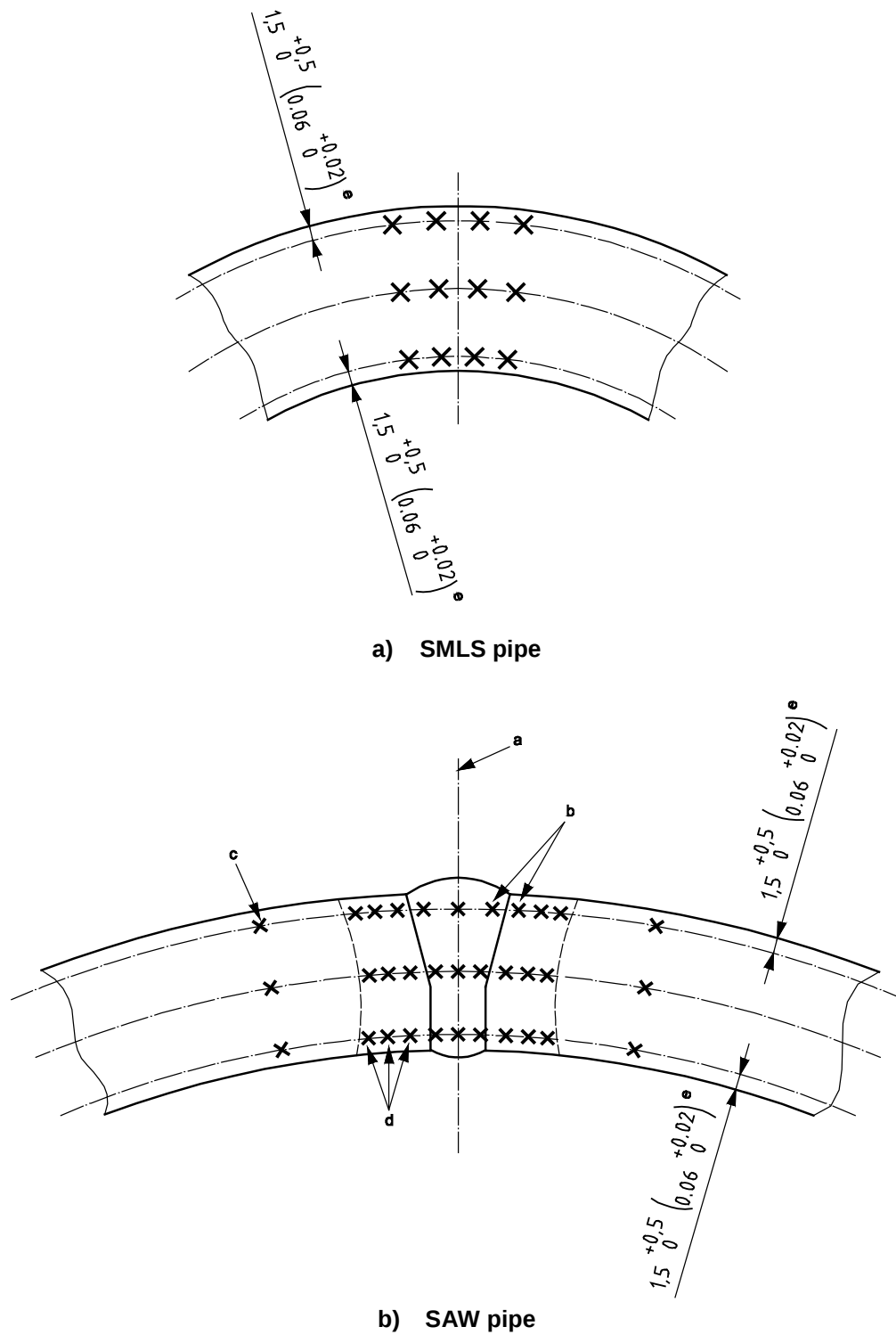
Figure N.1—Location of Hardness Tests
